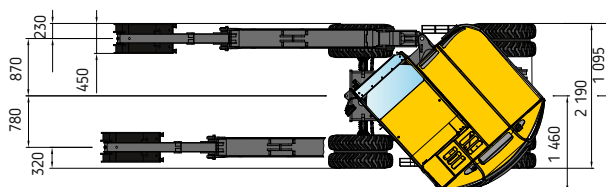
Abb. 1 : Aushub über die gesamte Breite der Maschine
